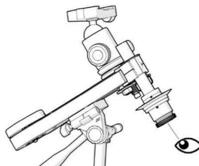
Imagen 3: así se alinea la montura MiniTrack con el polo norte celeste
